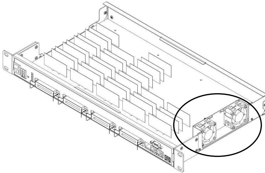
Fig. 6 - Fan location
